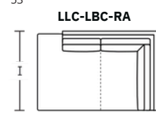
H: Grand 87", Studio 79", Micro 71" I: Grand 57", Studio 57", Micro 53"
