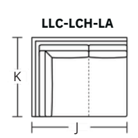
J: Grand 69", Studio 61", Micro 53" K: Grand 57", Studio 57", Micro 49"
