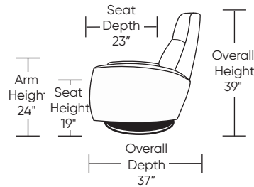
EVA-RV5-ST
